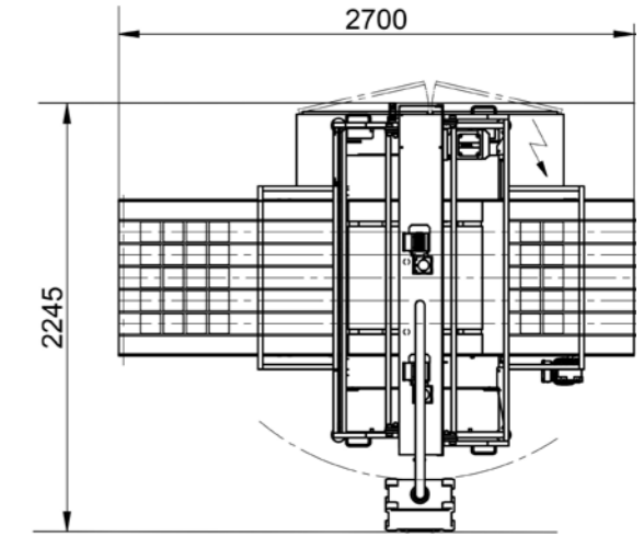
Unverbindliche Angebotszeichnung.
